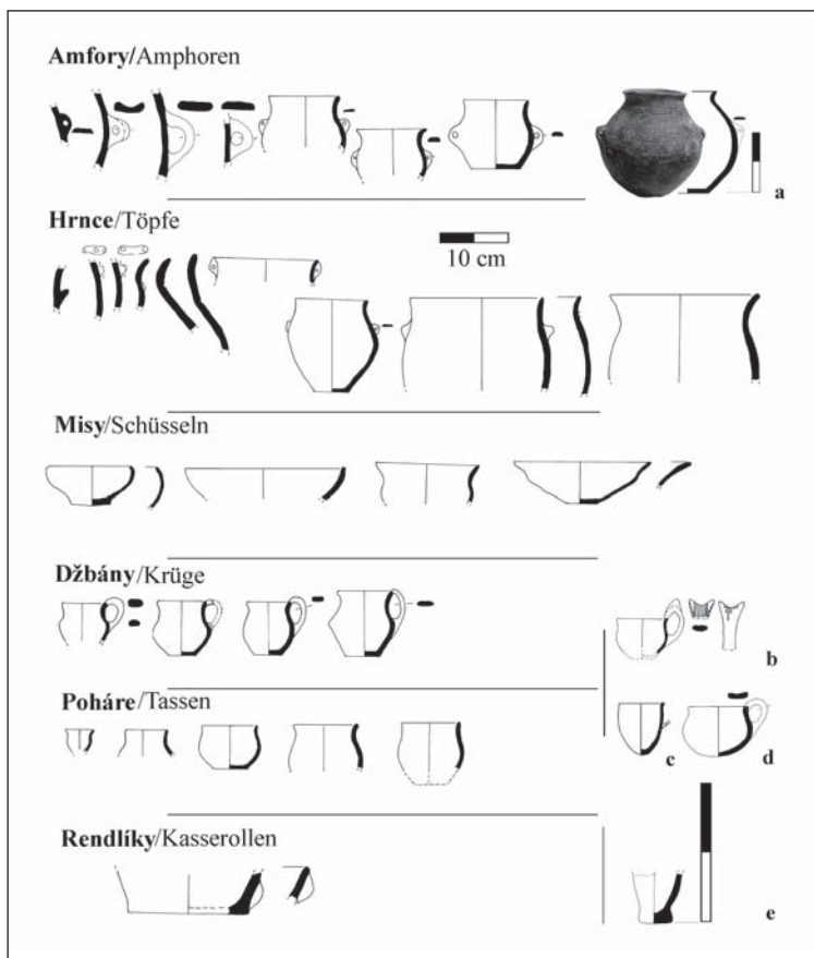
■ OBR. 3 Kočín – jevišovická kultúra. Tabuľka základných tvarov keramiky. Mierky uvedené.
